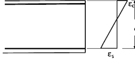
Şekil 1. Betonarme bir kesitte dönme ve birim uzamalar
